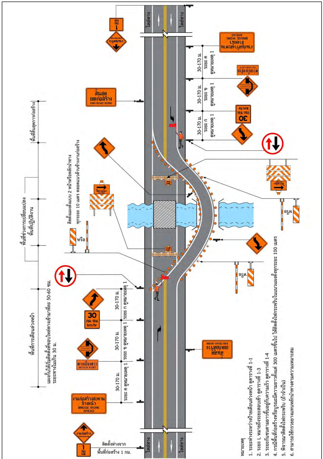
รูปที่ 4-13 การติดตั้งป้ายในงานก่อสร้าง/งานบูรณะ ชุตทางเปี้ยวหรือสะพานเปี้ยว สำหรับ 1 ช่องจราจร
