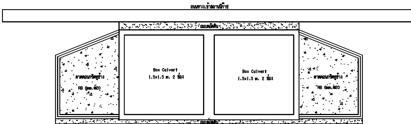
มุมมองทางระบายน้ำ หน้ากว้าง 4 เมตร
