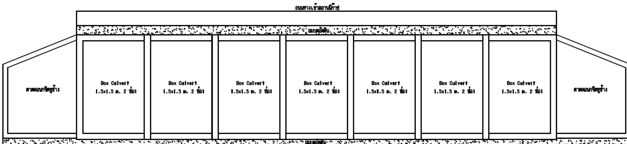
มุมมองด้านข้างทางระบายน้ำ หน้ากว้าง 7 เมตร
