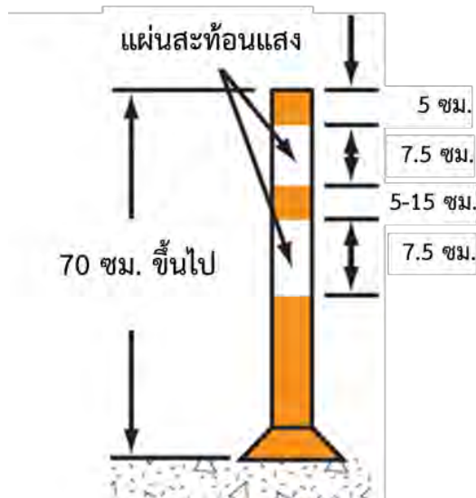
รูปที่ 3-2 อุปกรณ์จราจรประเภทเสาจราจรล้มลุก
