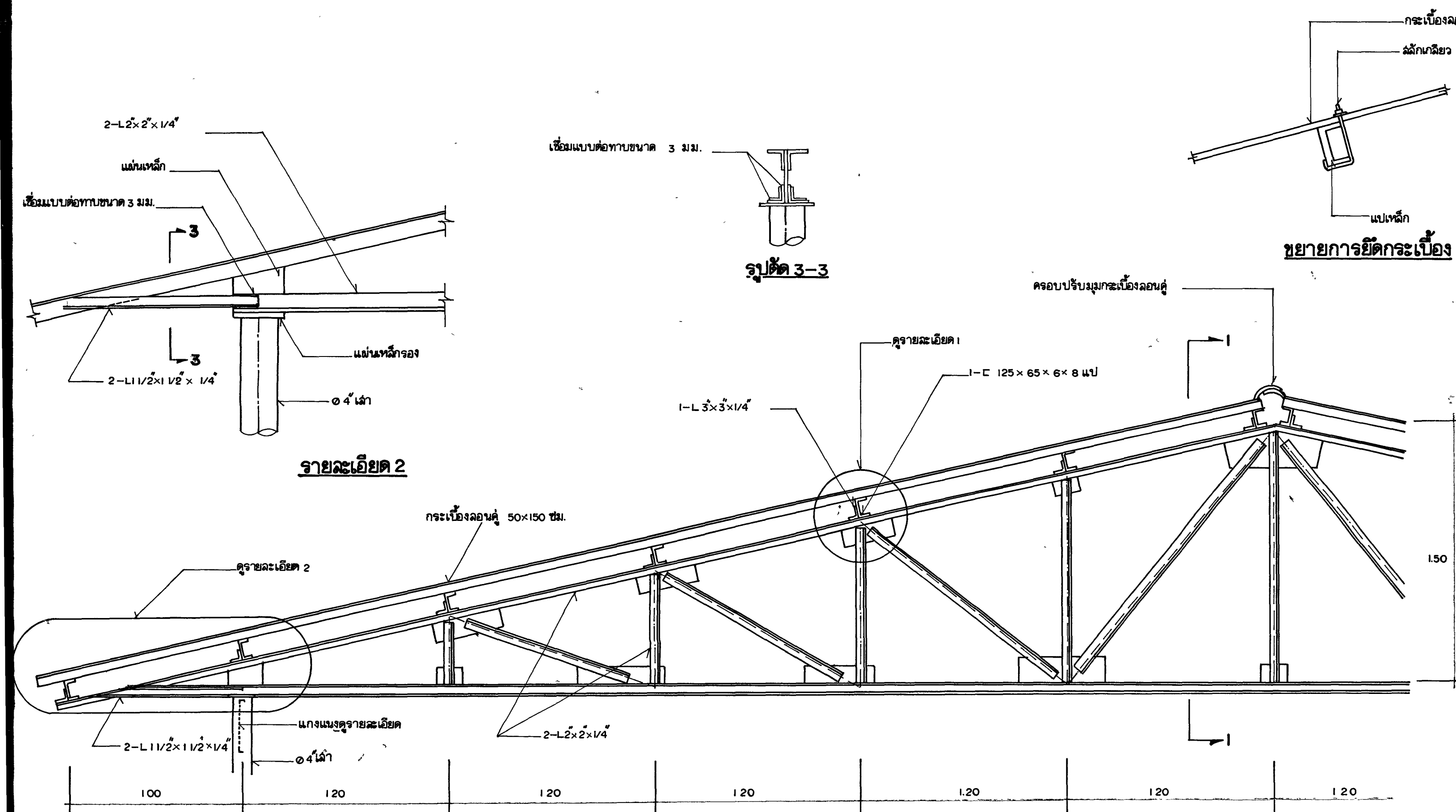
รายละเอียดโครงหลังคา 1:20
