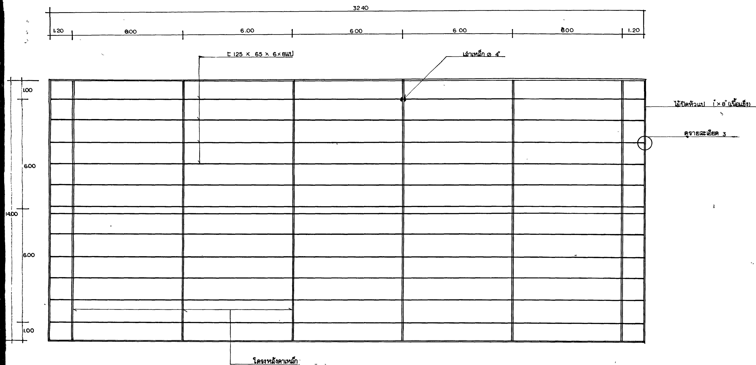
แปลนโครงหลังคา 1:100
