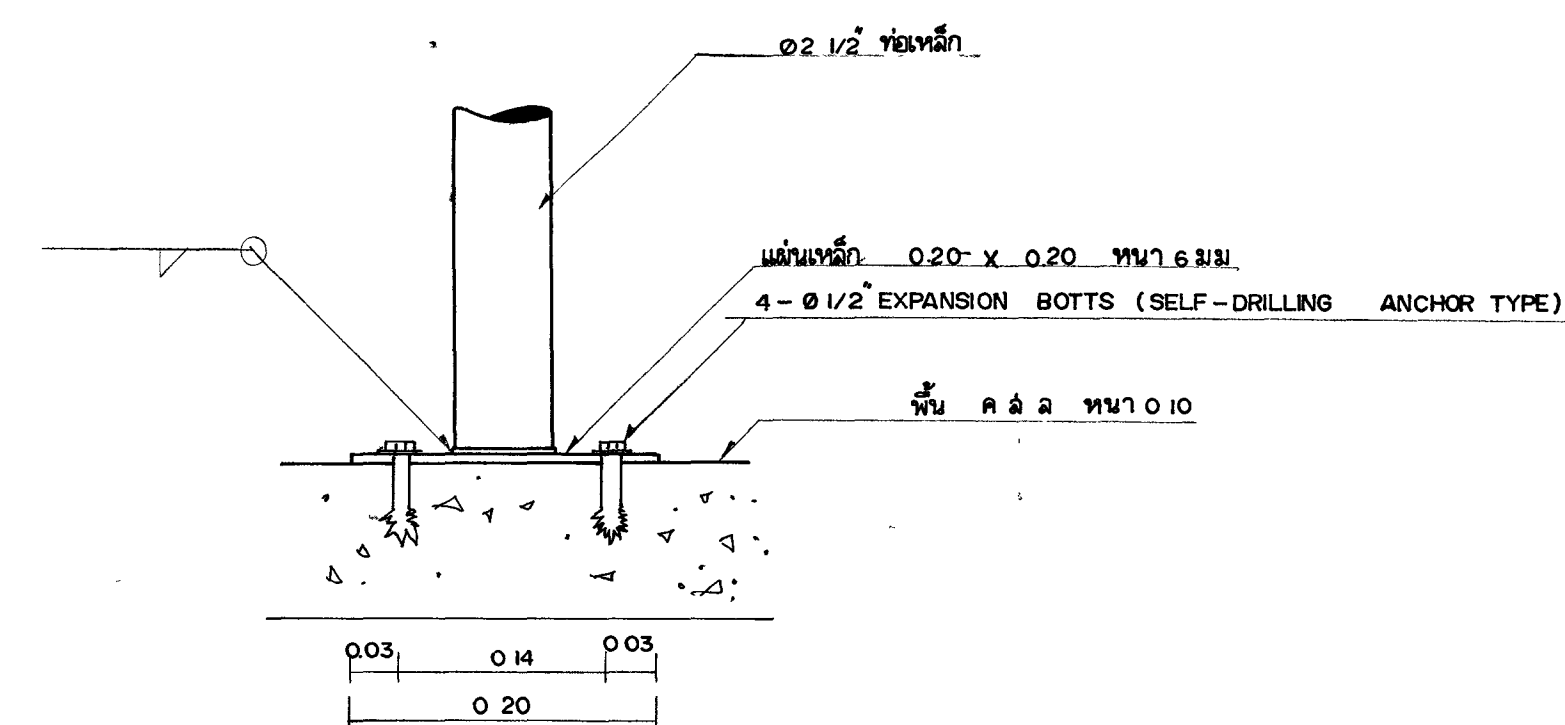
รายละเอียดการยึดต่อเหล็กกับพื้น ค.ฉ.ฉ. 1:5
