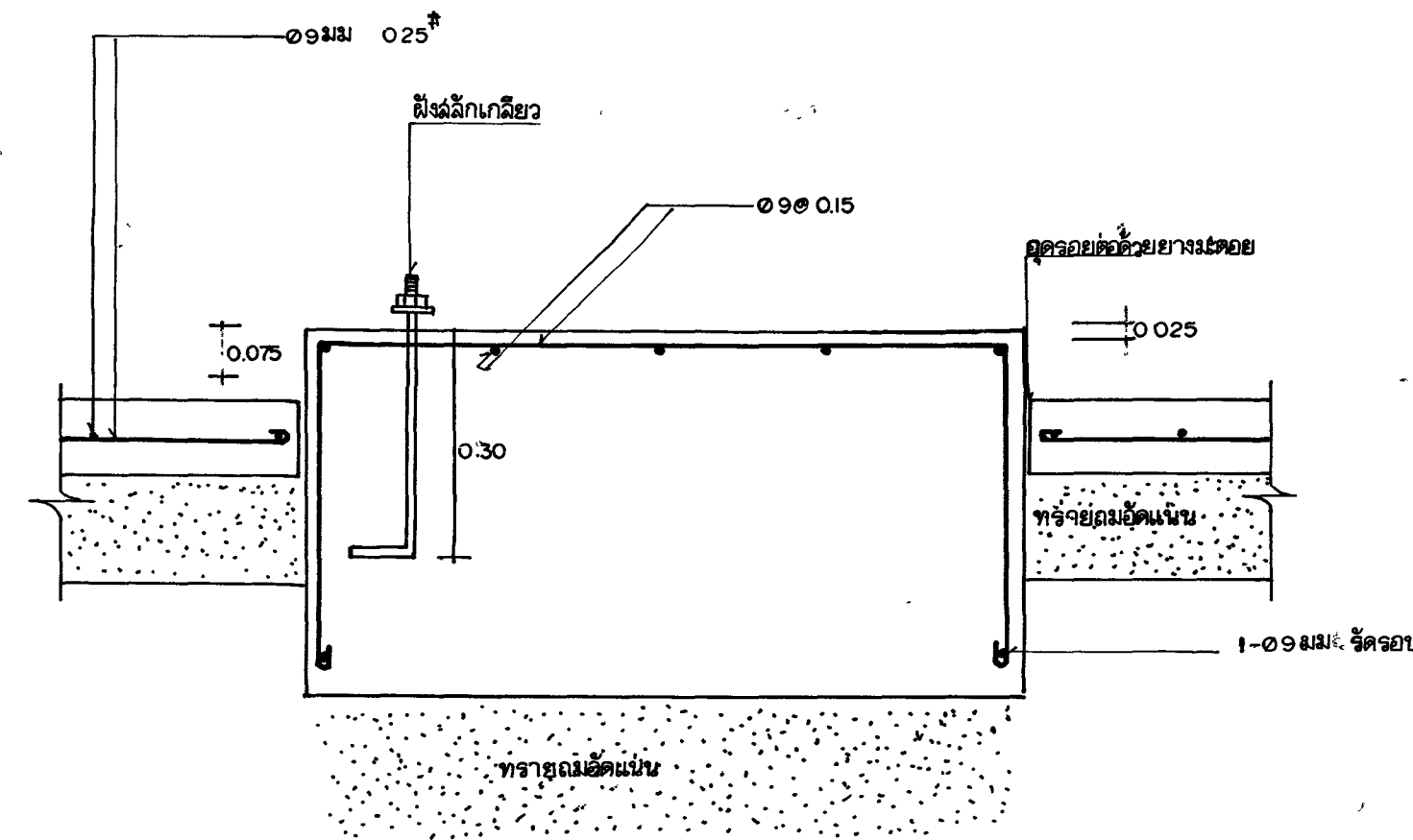
รูปตัดผ่านเครื่องขนาด 1.00 x 0.65 1:10
