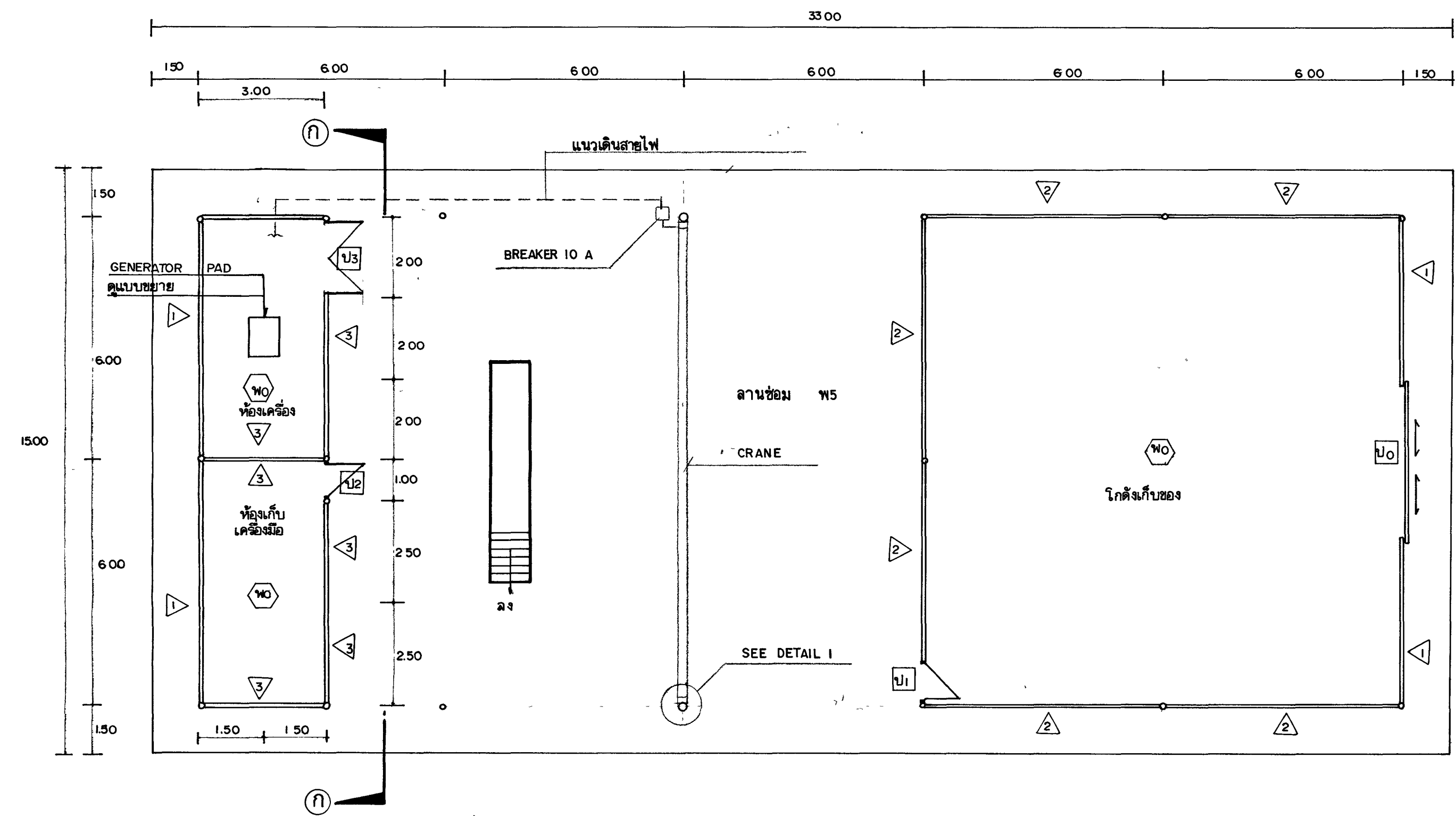
แปลนพื้นอาคารซ่อมบำรุงคลังพัสดุ 1:100
