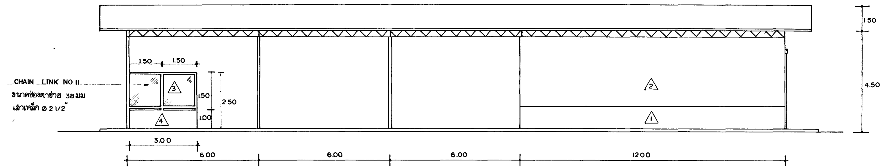
รูปด้านทิศใต้ 1:100
